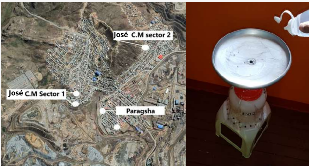
Sitios de monitoreo en Cerro de Pasco e instrumento de muestreo- Elaboración propia
